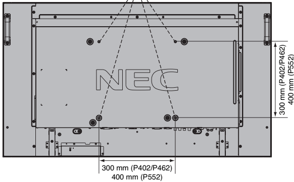
Interfejs montażowy VESA
