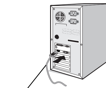
Przewód HDMI
