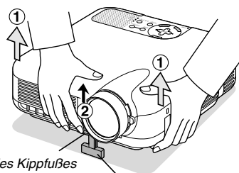
Einstellbarer Kippfuß
